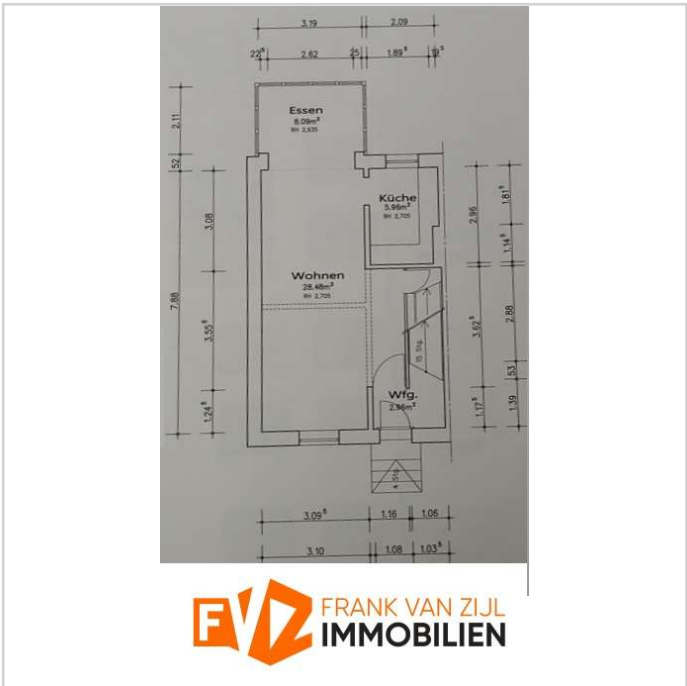
Grundriss Hochparterre
